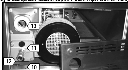
Вид сбоку 2-камерных машин серии POLAR при снятом кожухе
